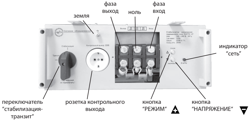
Рис. 5. Вид со стороны верхней панели стабилизатора (модели СНПТО-18, СНПТО-22, СНПТО-27)
