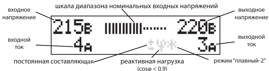
Рис. 9. Вид ЖК-индикатора в режиме плавного регулирования
